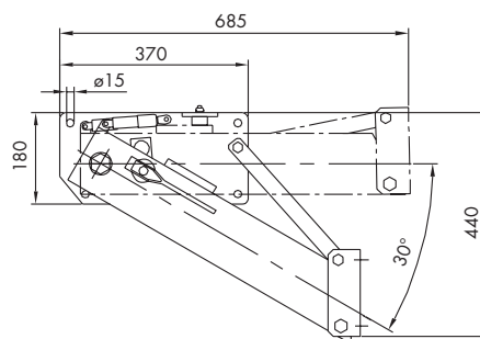
Ausf. Parallelogramm
