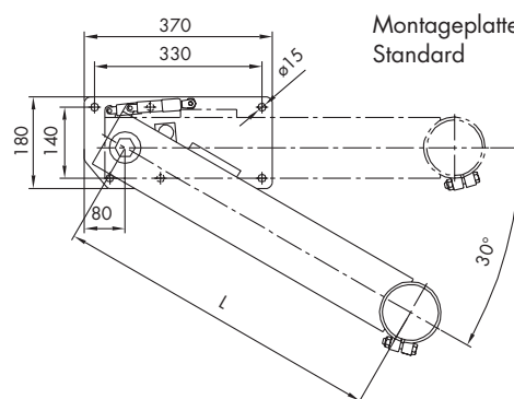
Ausf. Parallelogramm
